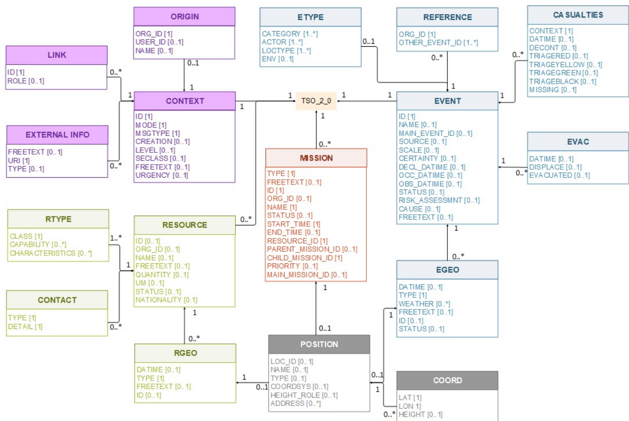
FIGURE 3.1 – Modèle de données EMSI 2015
