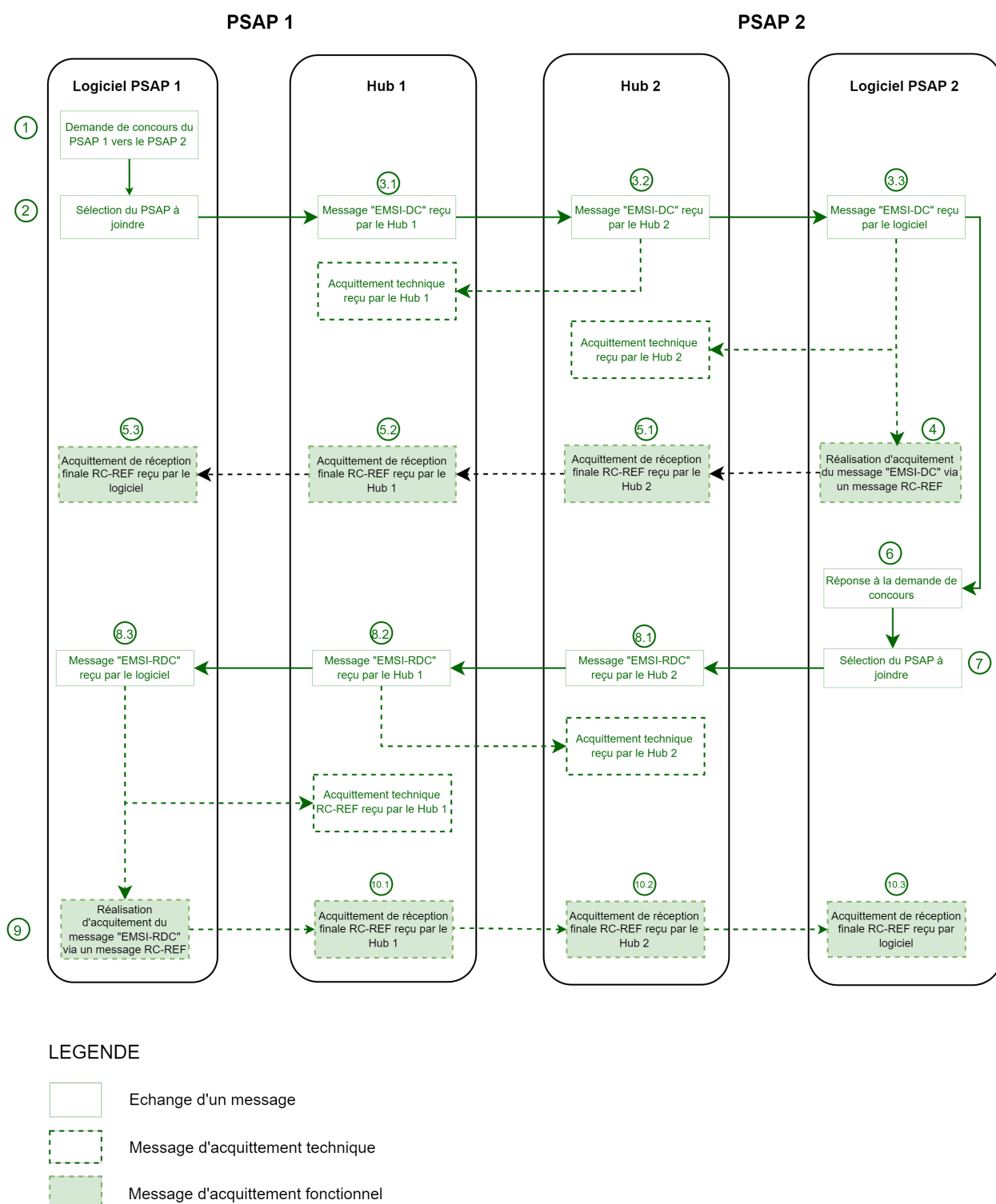
FIGURE 7.18 – Cinématique d'une demande de concours et réponse à la demande de concours
