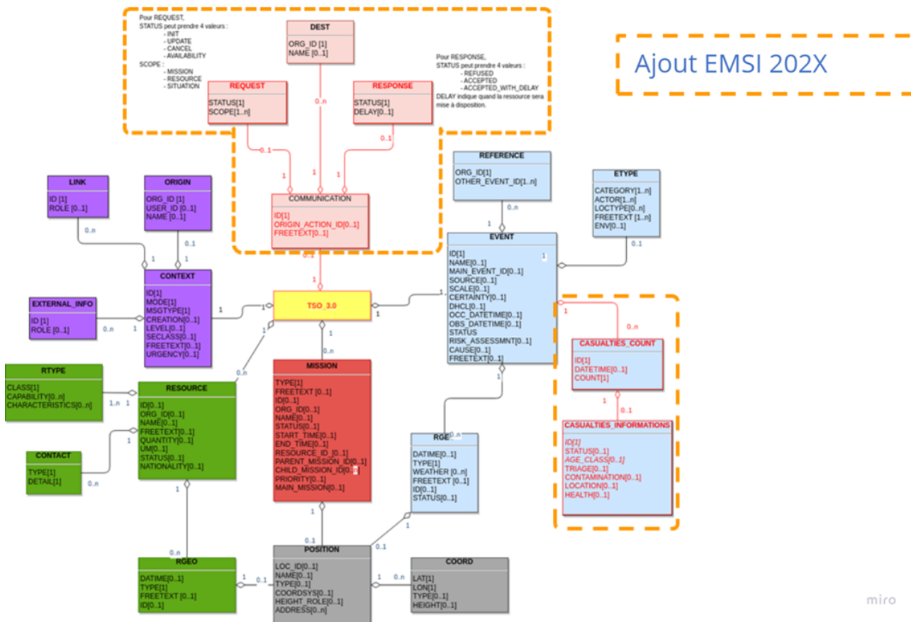
FIGURE 7.22 – Modèle de données de l'EMSI 202X
