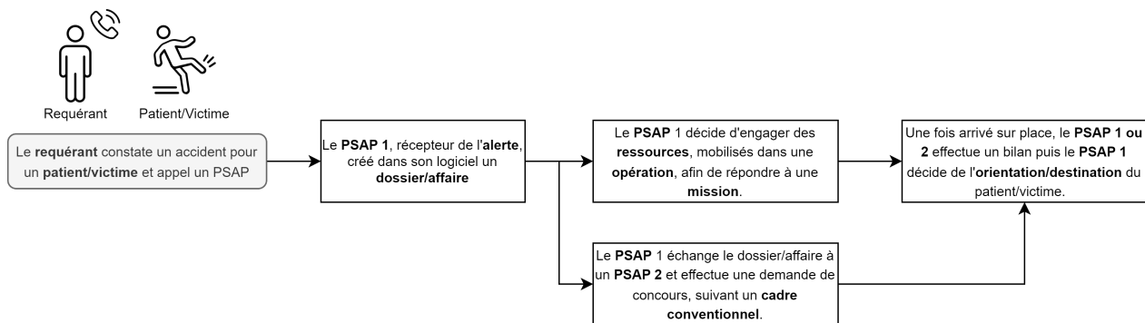
FIGURE 2.2 – Étapes métier de gestion d'une alerte
