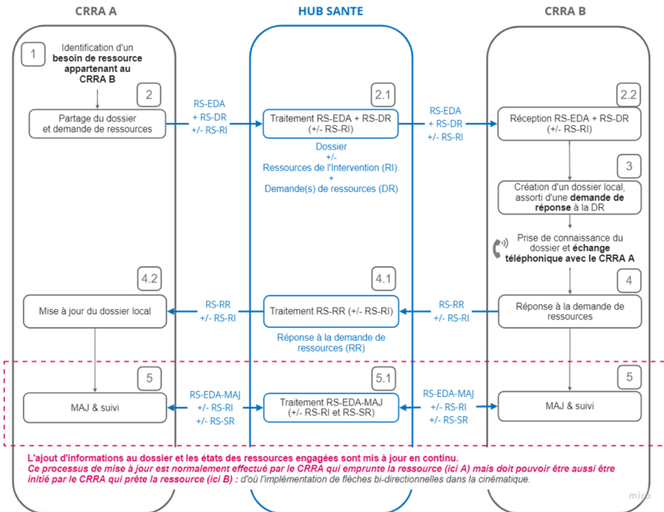
FIGURE 4.17 – Cinématique cas passant - demande de ressources
