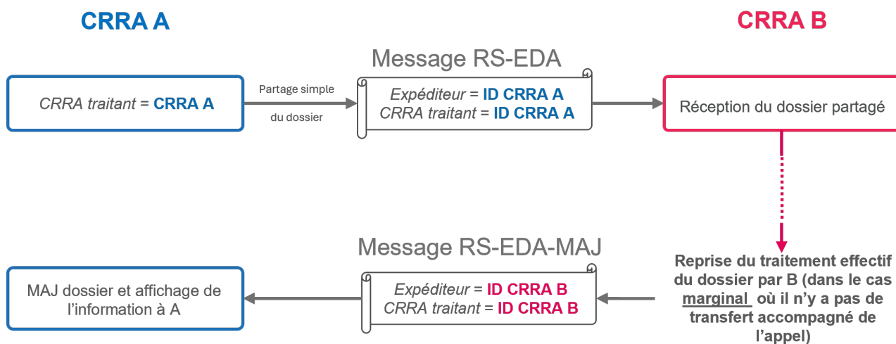
FIGURE 4.13 – Process d'utilisation de la donnée "CRRRA traitant" en l'absence de transfert d'appel
