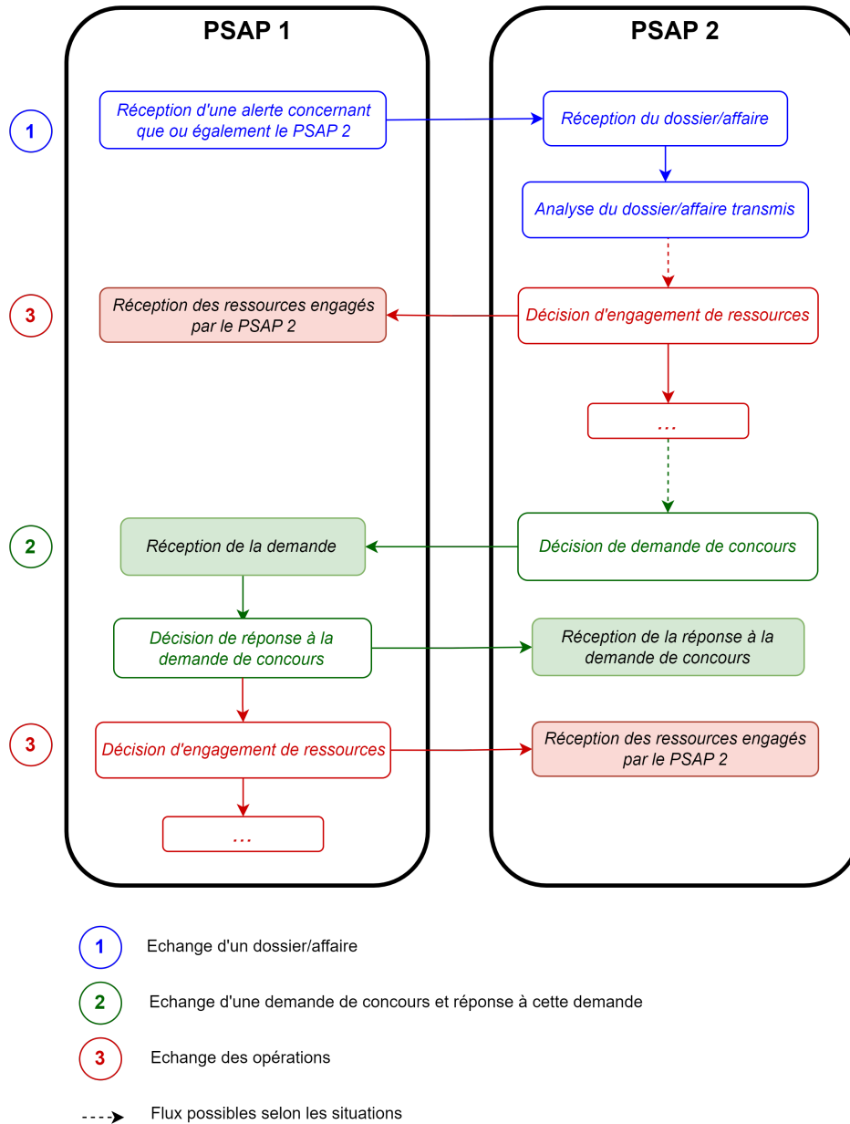
FIGURE 7.8 – Illustration du séquençage de blocs fonctionnels dans un cas d'usage
